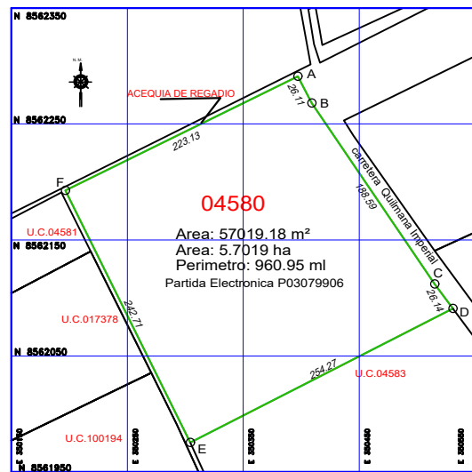
PLANO PERIMETRICO ESCALA : 1/2000
